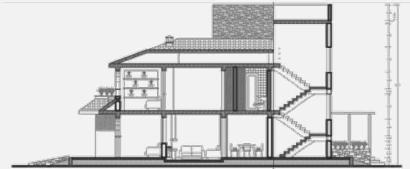
Corte 1-1
