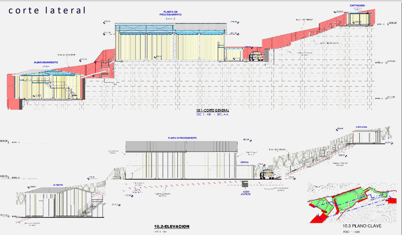
Elevación lateral
