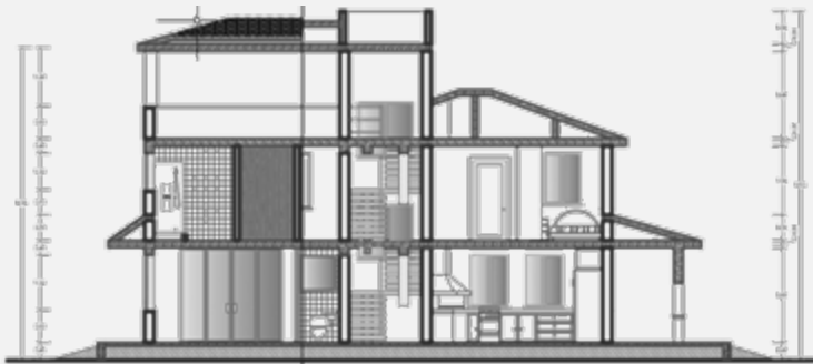
Corte 2-2
